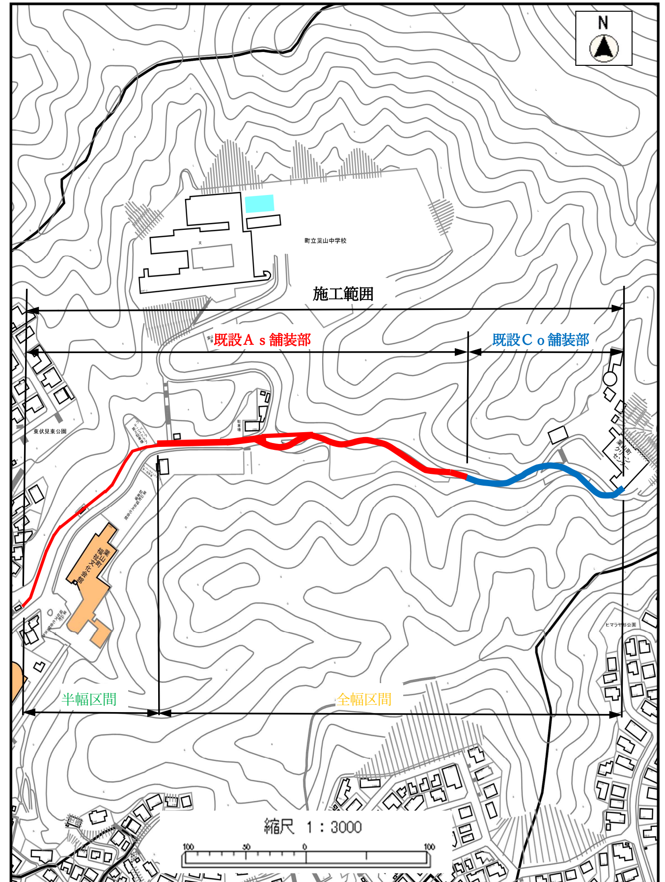
【施工範囲・施工区分図】
