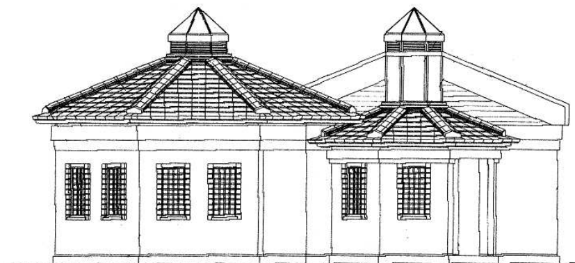
西側立面図
